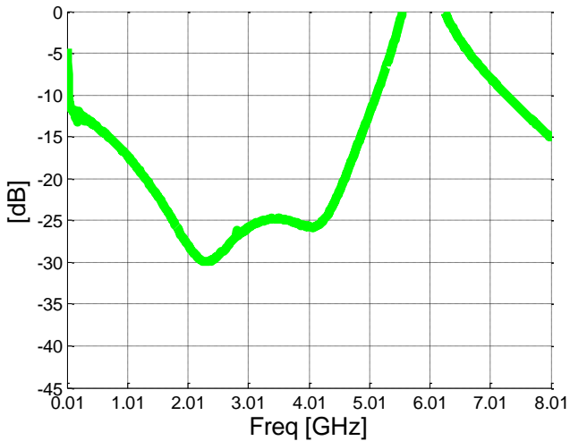
CMRR
